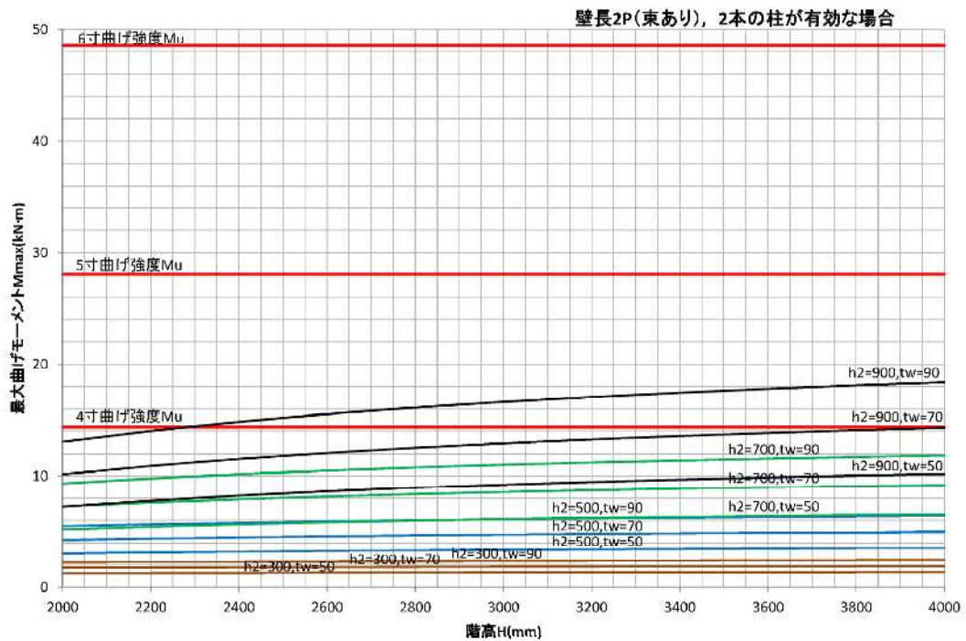
付図4 小壁が取りつく柱の折損に対する検討 (2本の柱が有効な場合(東あり)、2P)
