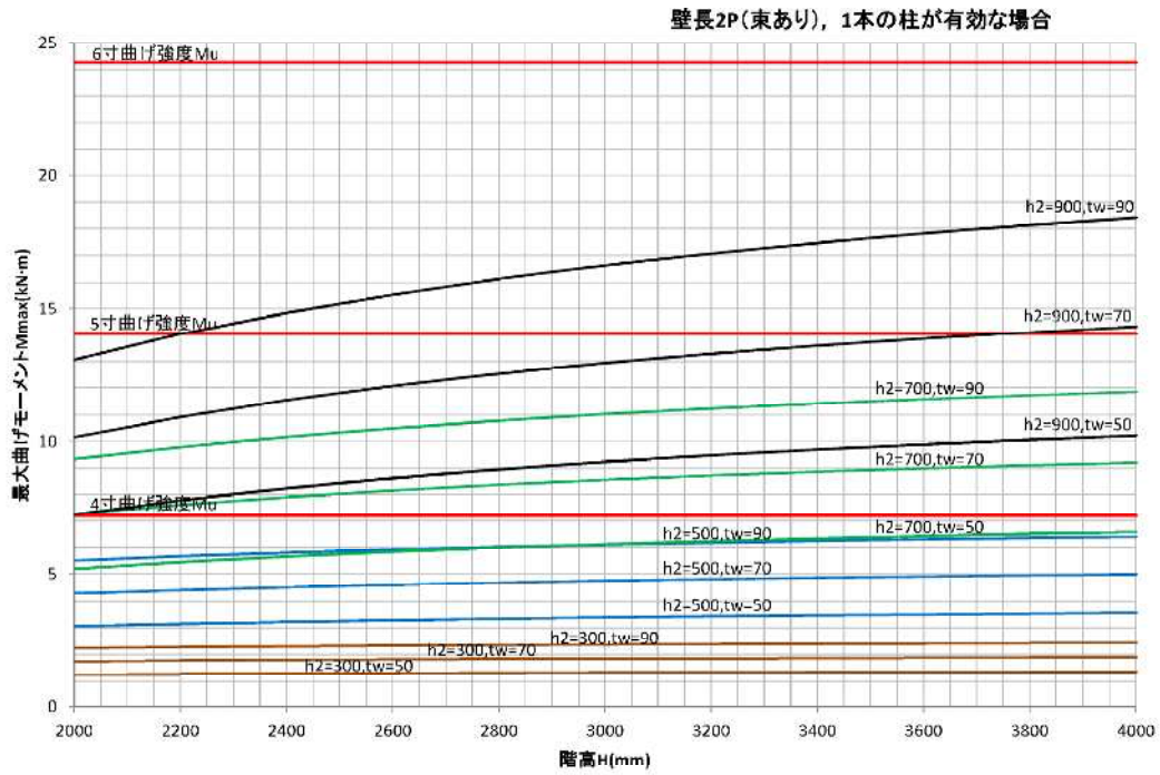
付図3 小壁が取りつく柱の折損に対する検討 (1本の柱が有効な場合(東あり)、2P)
